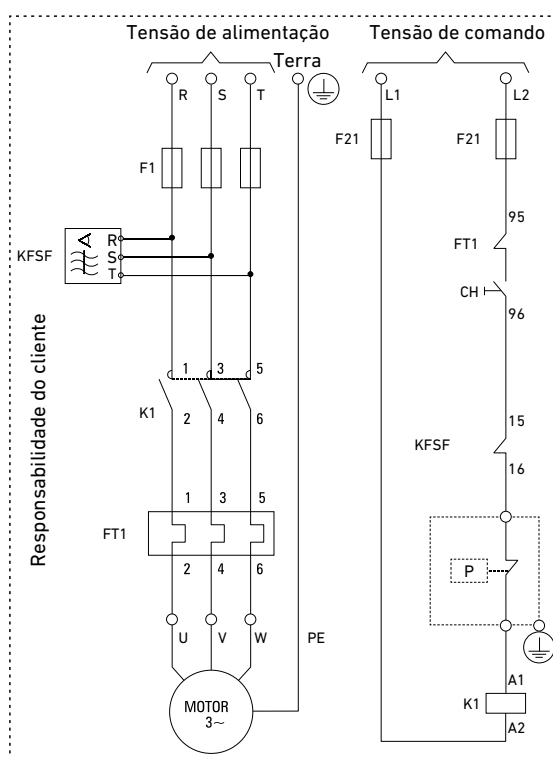
MOTORES TRIFÁSICOS - PARTIDA DIRETA
